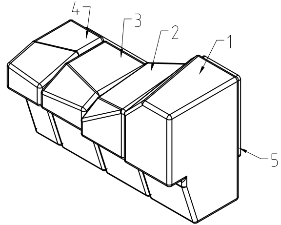
充磁方向示意图
