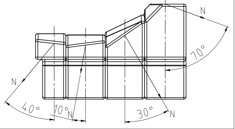
充磁方向示意图
